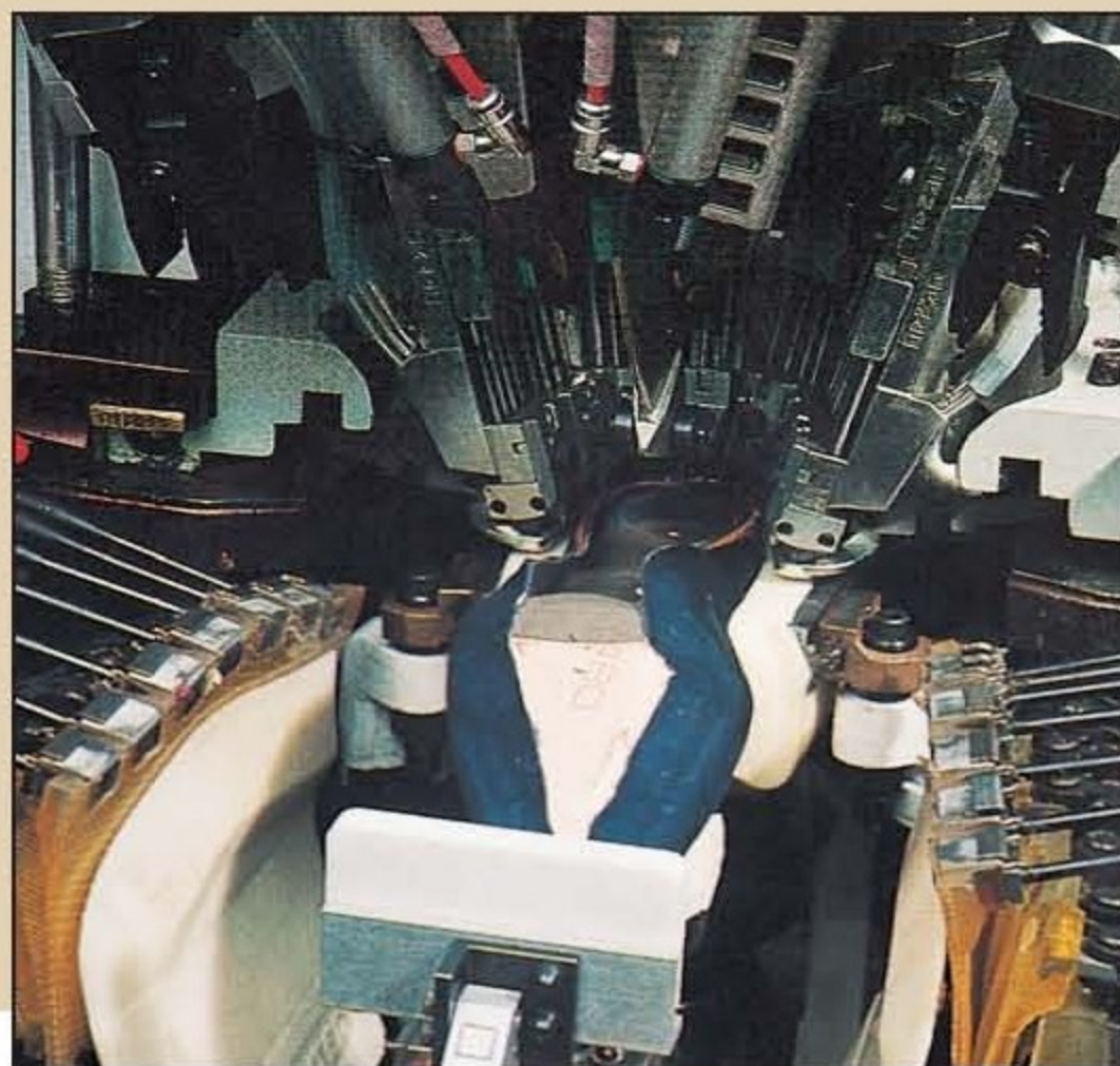
Fase di bloccaggio scarpa con riconoscimento automatico lunghezza scarpa. Phase of shoe blocking with shoe size automatic recognition. Fase de bloqueo del zapato con reconocimiento automatico largo del zapato. Phase de blocage chaussure avec reconnaissance automatique longueur chaussure.
