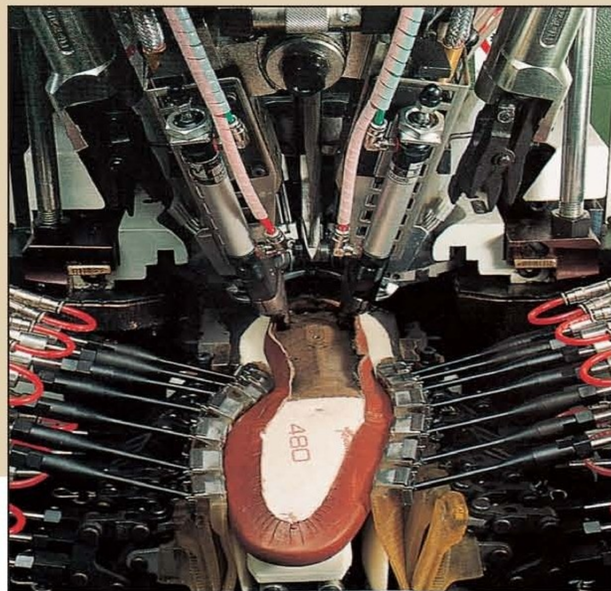
Fase di iniezione termoplastico nella boetta. Phase of hot melt injection in the heel seat. Fase de inyeccion de termoplastico en el talon. Phase d'injection thermoplastiques dans l'emboitage.
