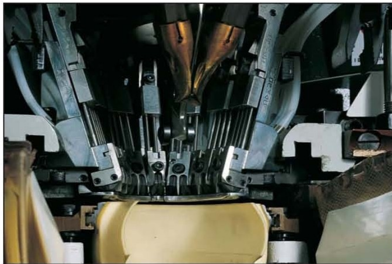
Piastre con posizione programmabile in apertura-chiusura e destro-sinistro. Wipers with programmable position opening-closing and left-right. Placas de montaje con posicion programable en abertura-cierre y derecho-izquierdo. Plaques avec position programmable en ouverture-fermeture et droit-gauche.
